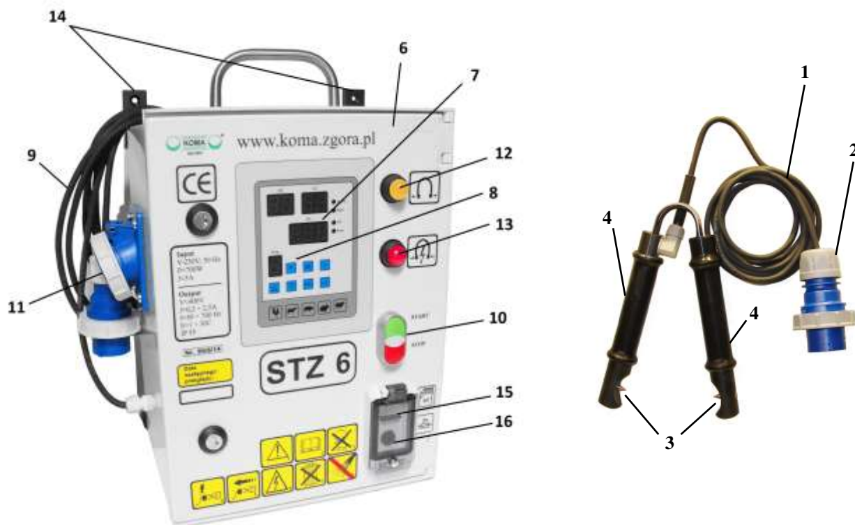
Rys.1 Urządzenie do głuszenia zwierząt STZ 6.
